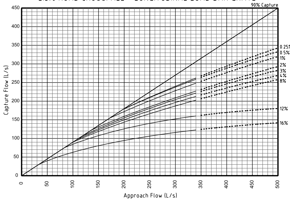
3% ROAD CROSSFALL - LONGITUDINAL LOAD BAR GRATE
