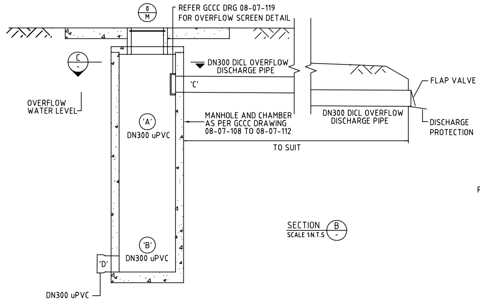
SECTION A SCALE 1:N.T.S.
